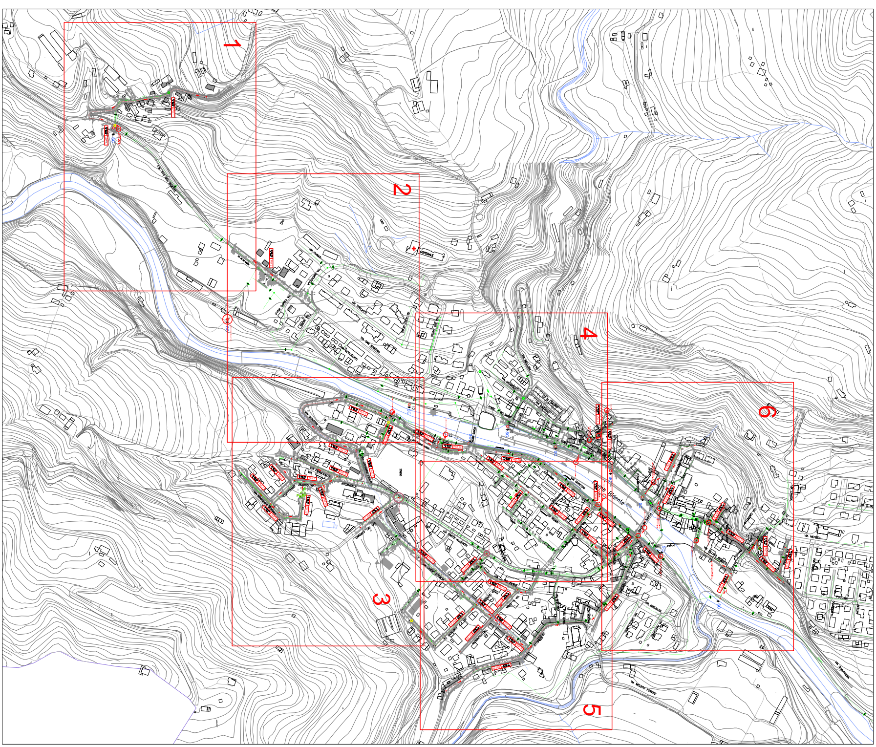
QUADRO D'INSIEME SCALA 1:500
